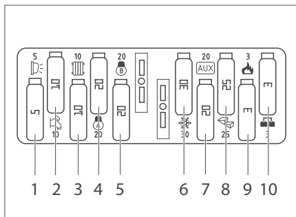
Bild 41 12-Volt-Sicherungen in der Modulbox (Abb. ähnlich)
