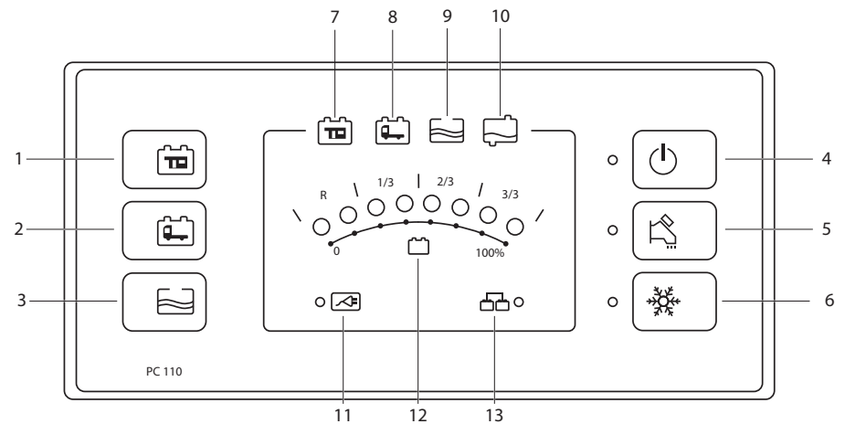
Bild 58 Control-Panel (PC110-HE)
