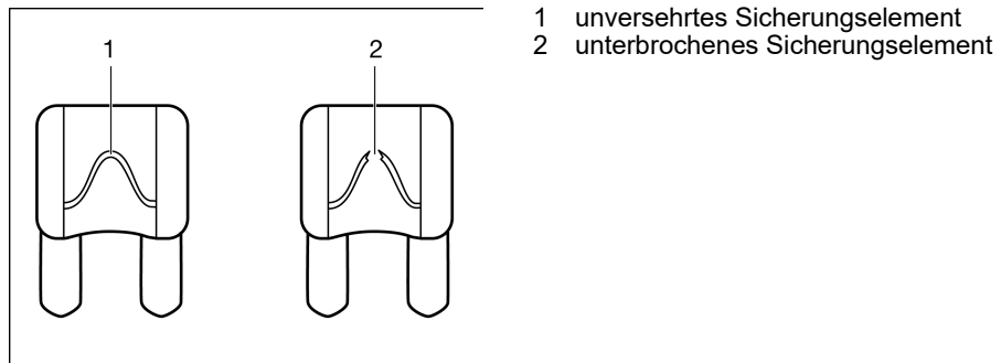
Bild 52 12-V-Sicherung
