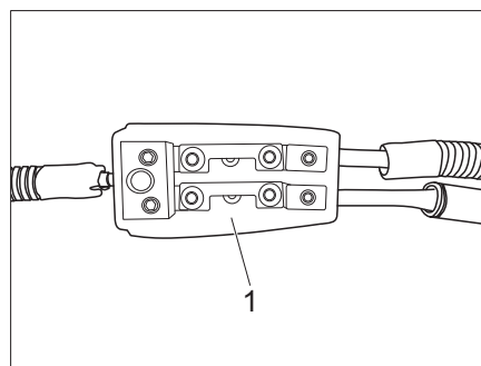
Bild 53 Sicherungen an der Wohnraumbatterie
