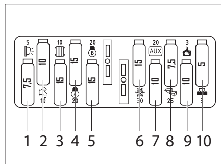
Bild 55 12-Volt-Sicherungen in der Modulbox (Abb. ähnlich)
